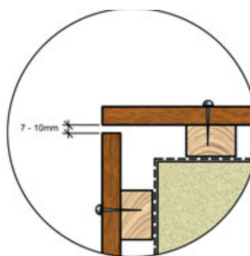
TEKENING B
