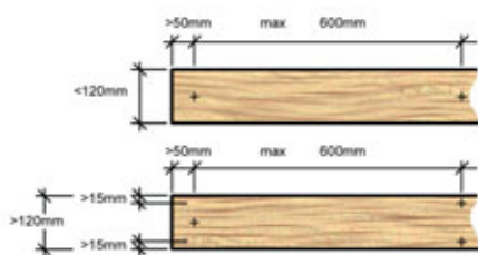
Maatvoering bevestigingspunten.
