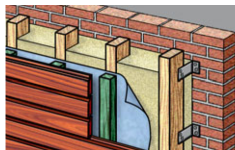
Opbouw gevelbekledingsconstructie bij een steenachtig binnenspouwblad, regelwerk verduurzaamd.
