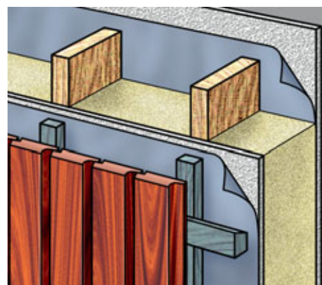
TEKENING A Een voorbeeld van een dubbel regelwerk.
